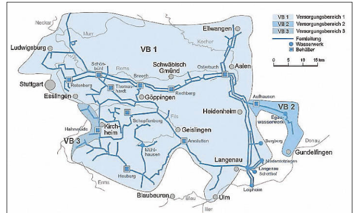
Das Fernleitungsnetz des Zweckverbands Landeswasserversorgung Foto: Landeswasserversorgung
