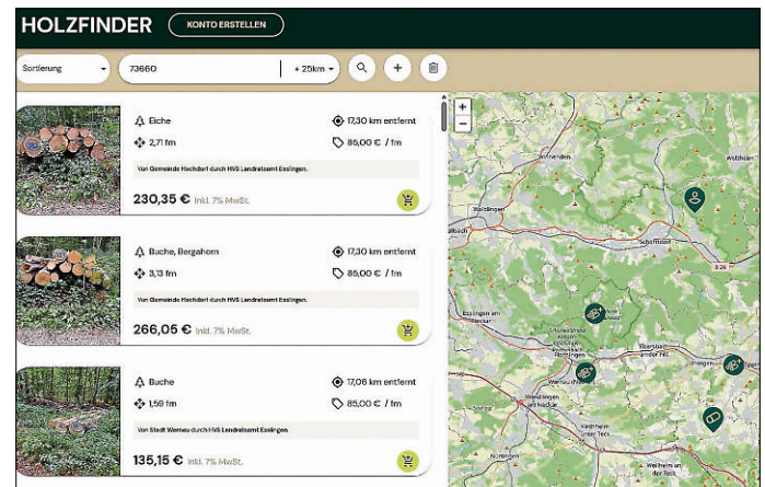
Screenshot Holzfinder
