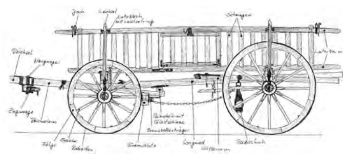
Bauzeichnung mit Beschriftung von Karlheinz Stegmaier Foto: Museumsarchiv
