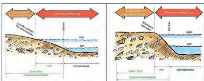
Abb. 3: Bemessung und Pflege des Gewässerrandstreifens (MW = Mittelwasserstand / MHW = mittleres Hochwasser) Grafik: W. Maerke/Büro im Fluss
